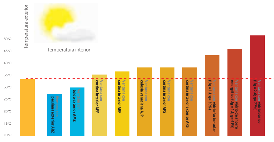
Temperatura máxima en el espacio bajo cubierta en un día caluroso dependiendo de los accesorios usados.
